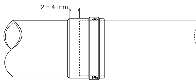
рис. 20 - Тепловое расширение
