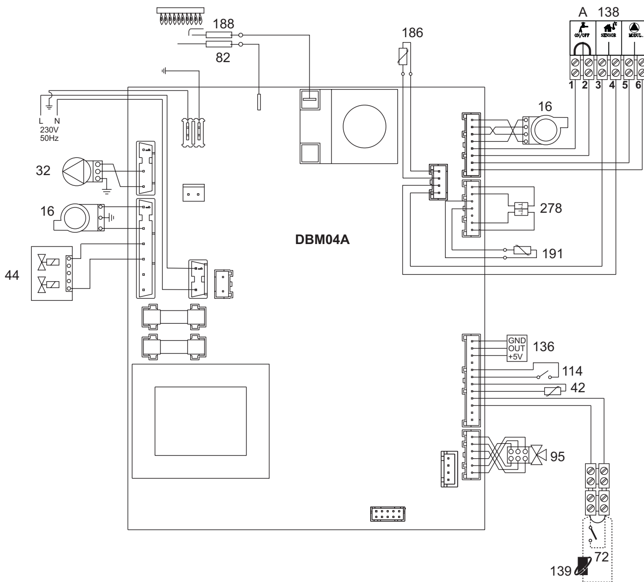
рис. 34 - Электрическая схема
