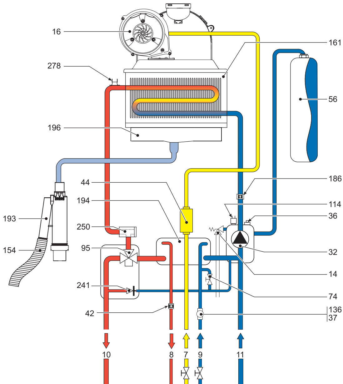
рис. 33 - Схема системы отопления и контура ГВС
