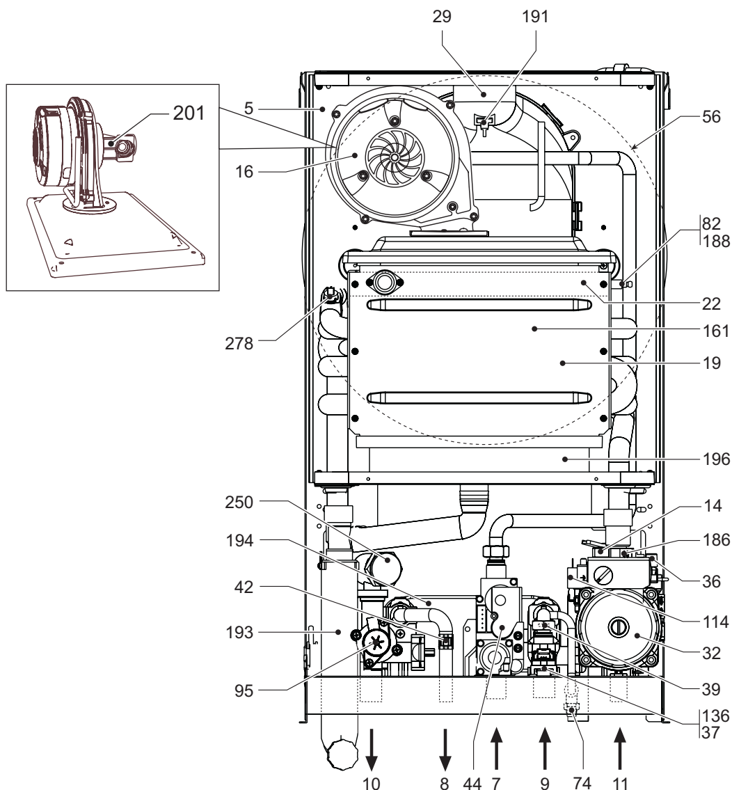
рис. 32 - Общий вид
