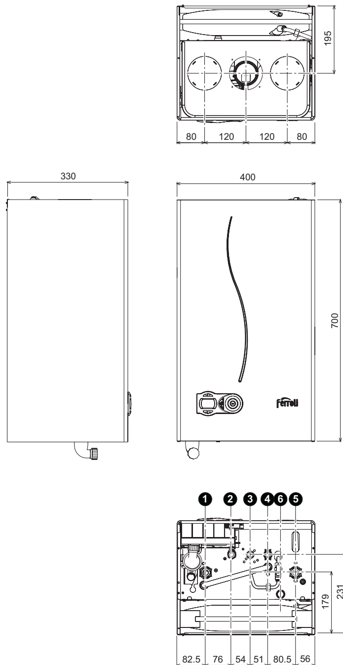
рис. 31 - Габариты и присоединения
